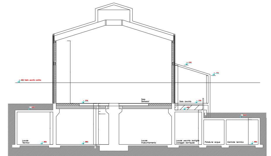
Sezione Schematica
