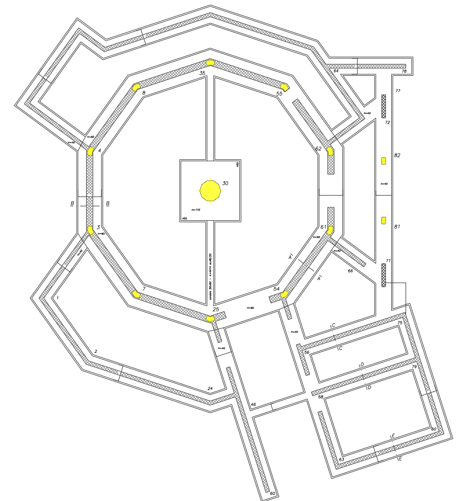
Pianta Fondazioni
