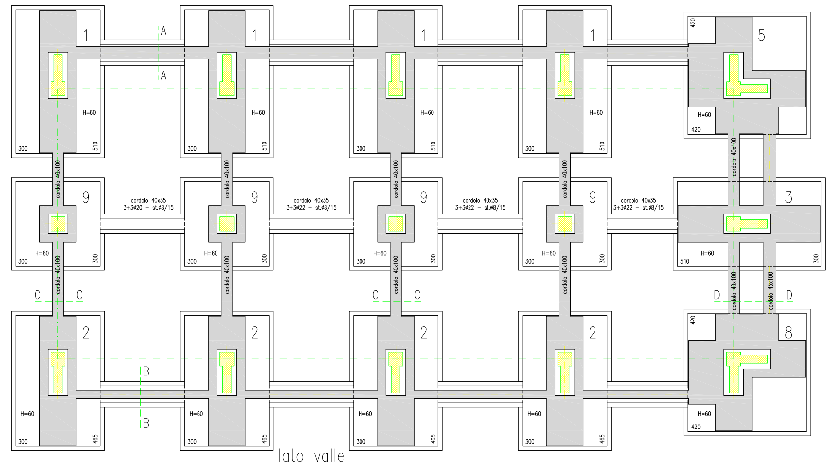
Pianta FONDAZIONI
