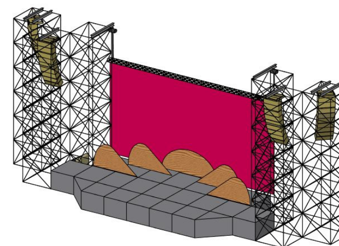
Figura 2: palco per evento "tutto Dante di Roberto Benigni"
