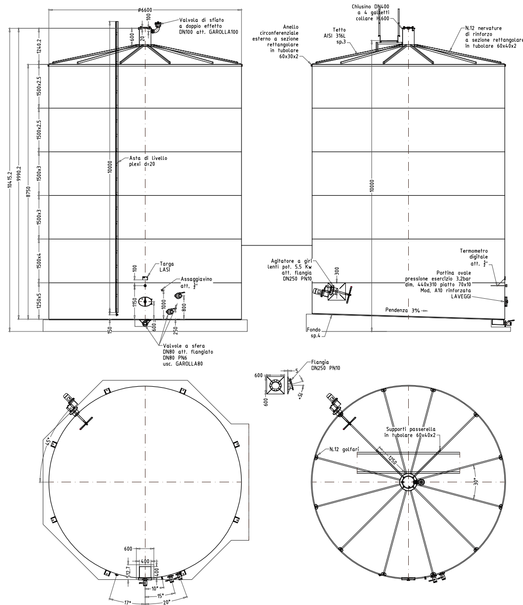
schemi silos: prospetti e piante
