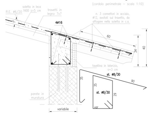
Particolare 1b: sezione cordoli di gronda
