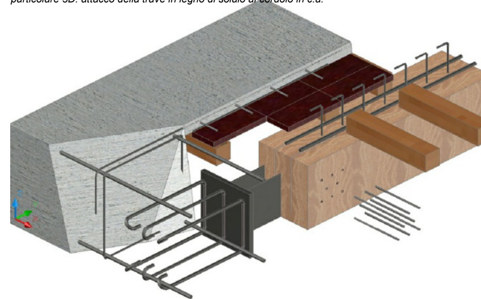
particolare 3D: attacco della trave in legno di solaio al cordolo in c.a.
