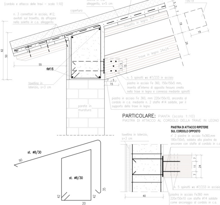
Particolare 1a
