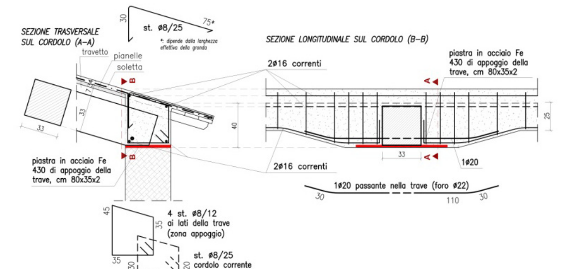
particolari strutture lignee (copertura), fabbricato principale
